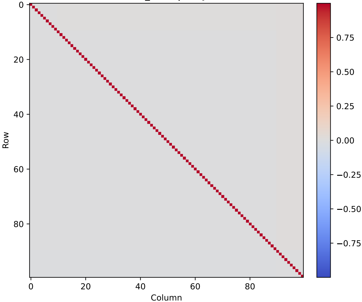
muon_zero | step 8
